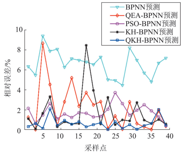
图6 空调负荷预测的相对误差
