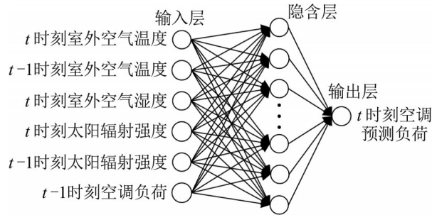
图3 BPNN空调负荷预测模型结构图
