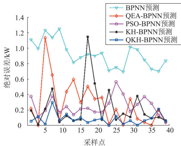
图5 空调负荷预测的绝对误差
