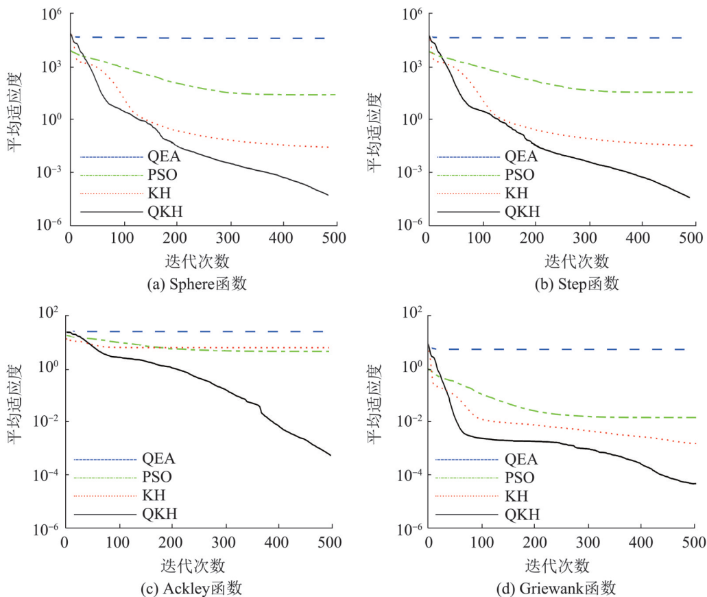
图2 测试函数平均适应度迭代曲线
