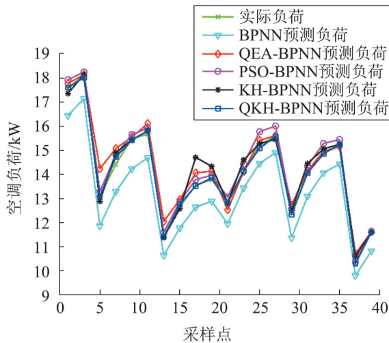
图4 空调负荷预测值
