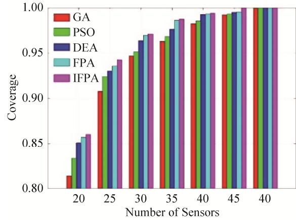
图15 节点数目与覆盖率
