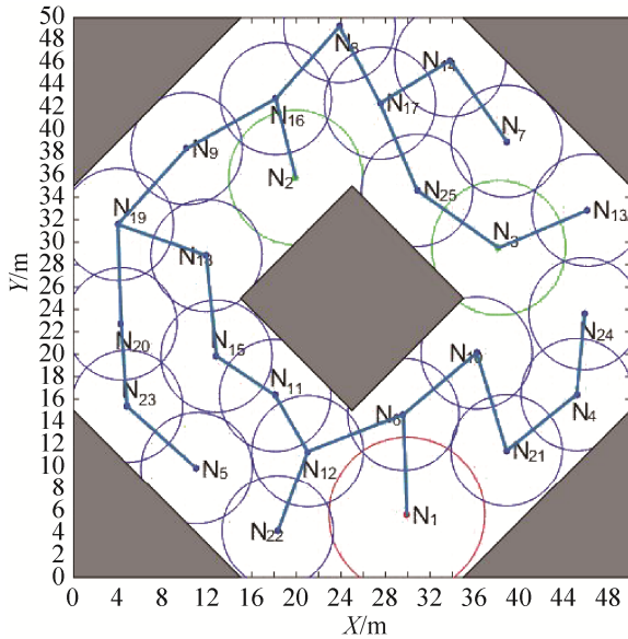
图13 最终部署图
