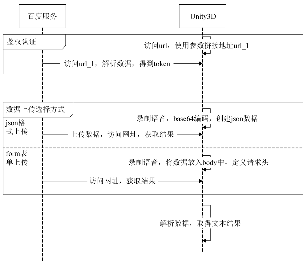
图3 语音服务与 unity 交互
