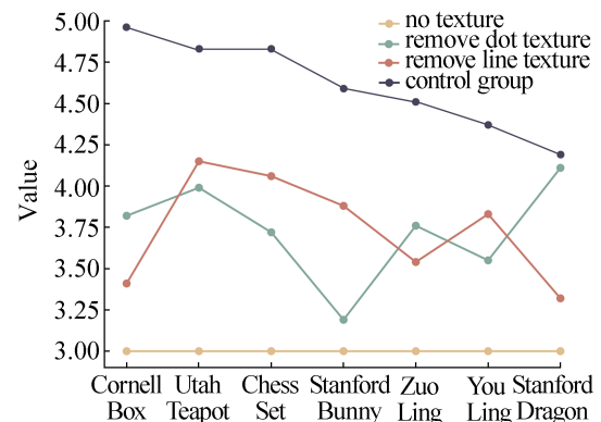
图 9 关于屏幕空间分区域渲染的消融实验结果 Fig. 9 Results of ablation experiment on screen space partition rendering
