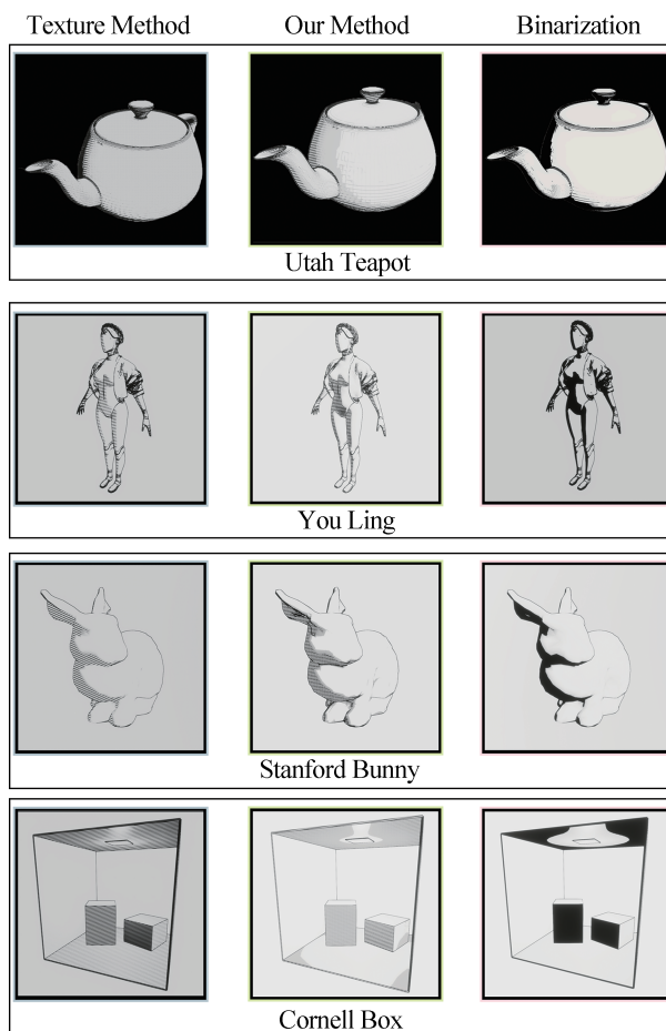
图 10 视觉效果对比实验中选取的部分渲染图片 Fig. 10 Some rendered images for visual effect comparative experiment
