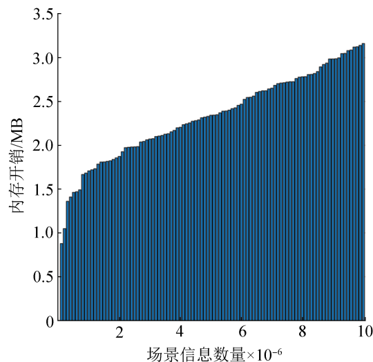
图6 渲染时内存消耗随场景信息变化
