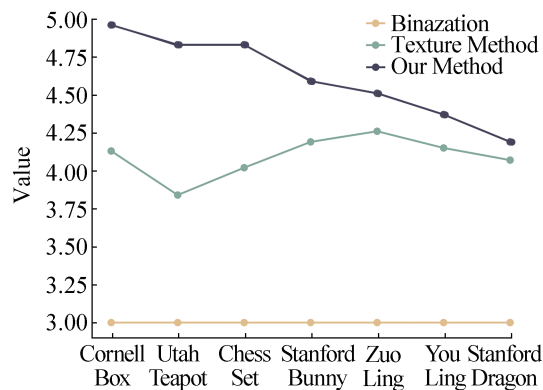
图 11 视觉效果对比实验结果 Fig. 11 Results of visual effect comparative experiment
